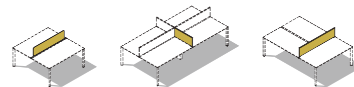
Screen W 100 / 140 / 160 / 180 D 1,8 - H 36 W 80 D 1,8 - H 32,9 / 37,1 W 160 D 1,8 - H 31,1 / 32,9 / 35,3 / 37,1
